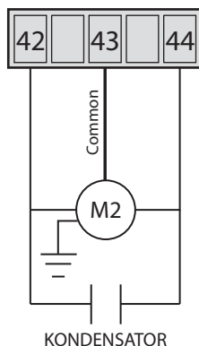
EINPHASIGE ELEKTROMOTOREN Versorgung
