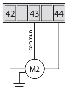
Alimentation MOTEURS ELECTRIQUES TRIPHASE
