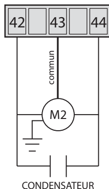
Alimentation MOTEURS ELECTRIQUES MONOPHASE
